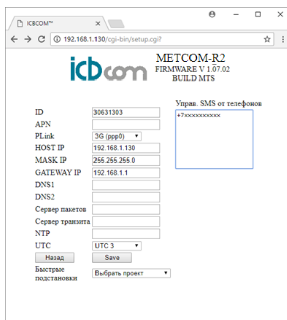
Рисунок 4. Вкладка « SETUP »
