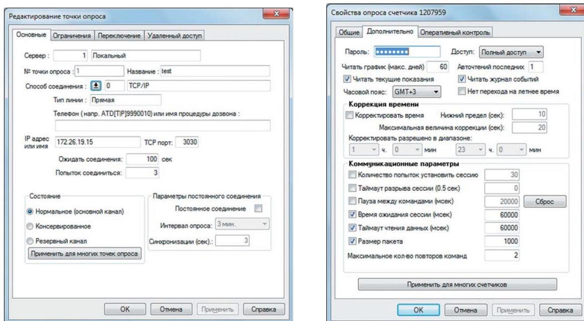
Рисунок 17. Настройки соединения
