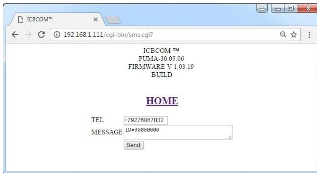
Рисунок 6. Вкладка “HOME” -> “SMS”
